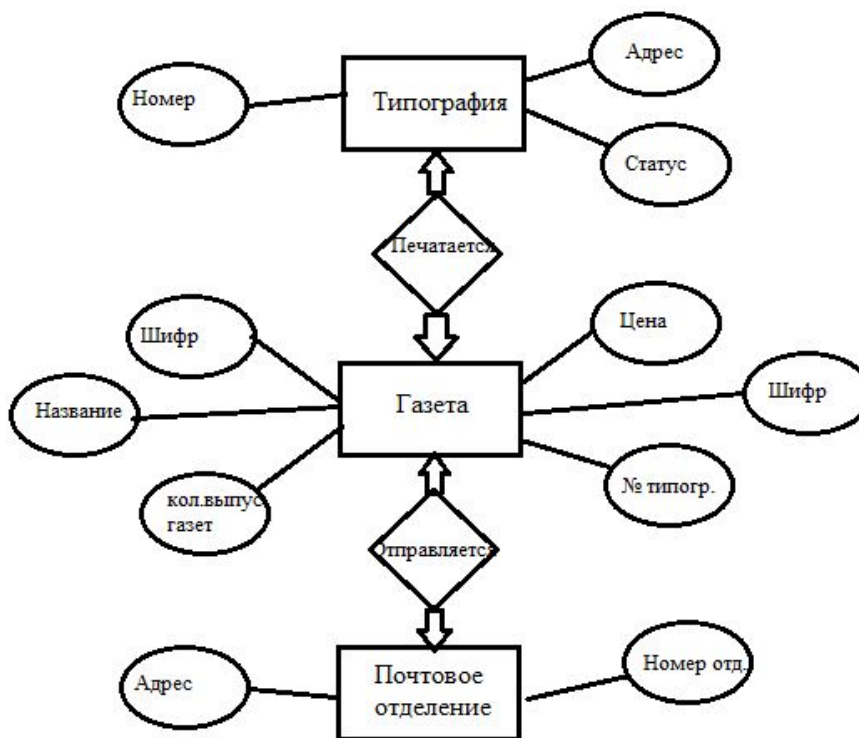
Рисунок 1 – ER-диаграмма модели базы данных
