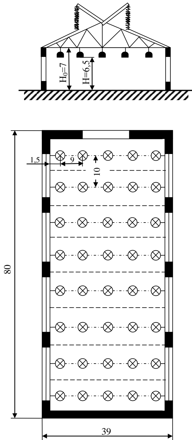
Рис.1. Литейный цех
